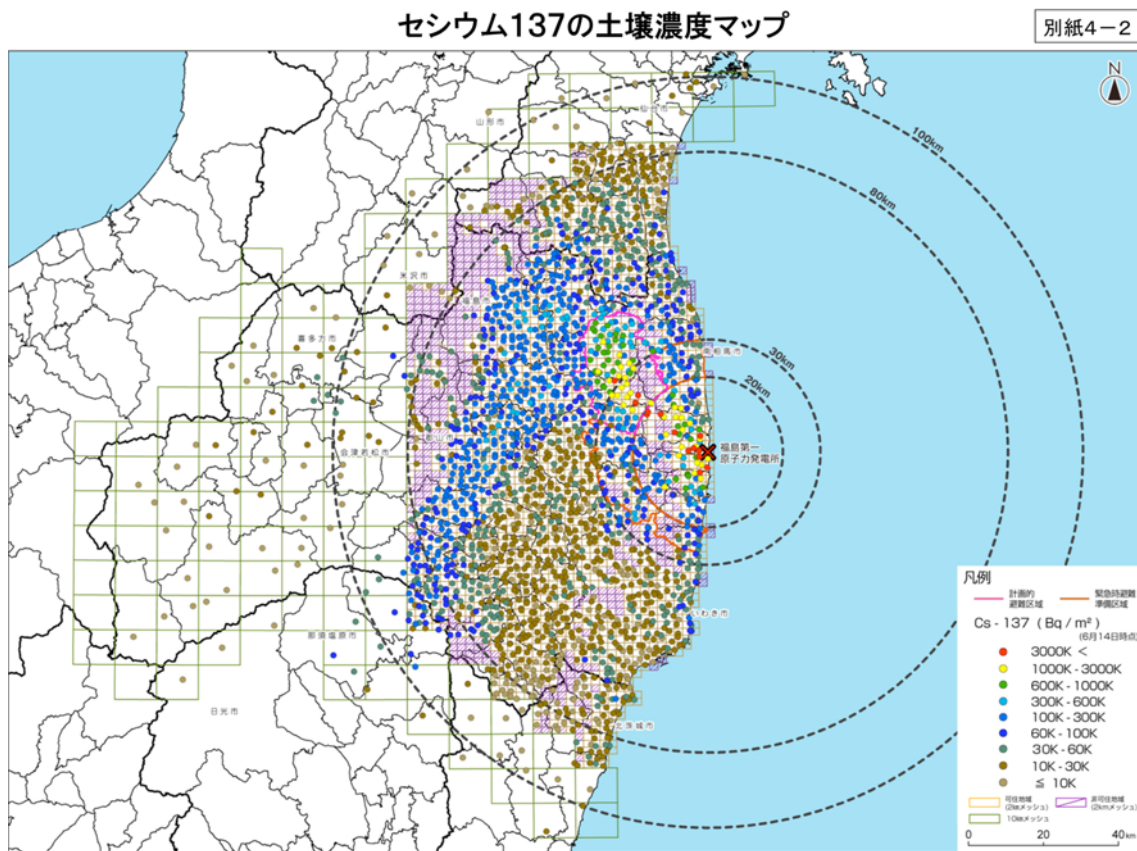
Césium 137 : carte de la contamination au sol
